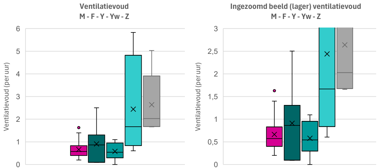
Figuur 18 a,b, Spreiding ventilatievoud in de 5 categorieën
