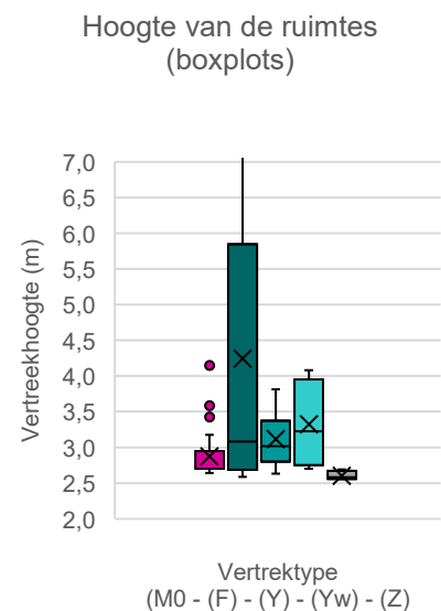
Figuur 9 Boxplots Vertrekhoogte (H in m) van de geïnventariseerde ruimtes in alle gebouwcategorieën
