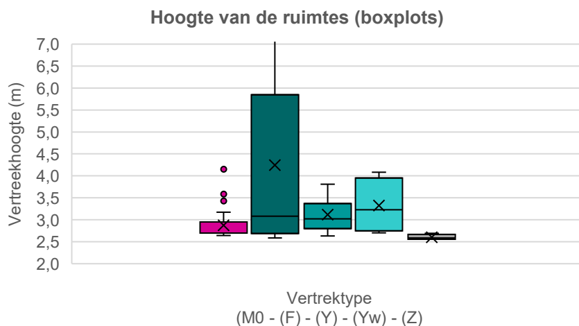
Figuur 22 Boxplots Vertrekehoogte ( H in m^1 ) van de geïnventariseerde ruimtes in alle gebouwcategorieën
