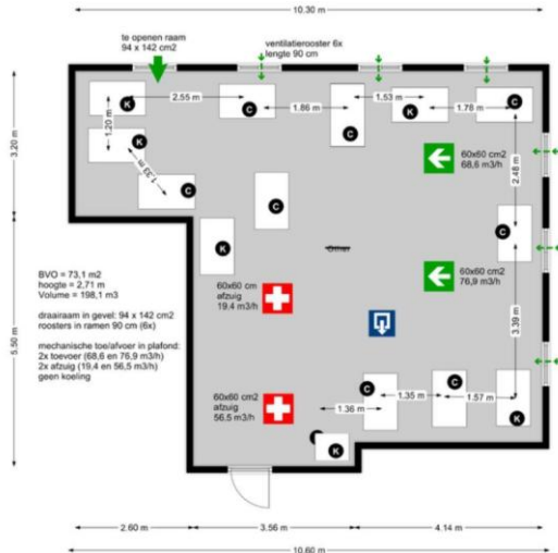
Figuur 1: Voorbeeld plattegrond met maatvoering, inrichting toestellen en locatie van ventilatievoorzieningen
