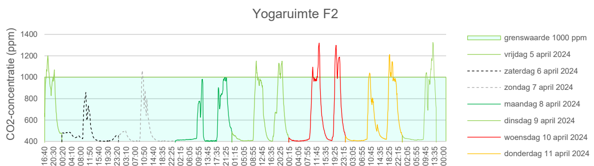
Figuur 31 De CO 2 -concentratie verloopt met pieken en dalen in een yogaruimte gedurende een week door lessen die of aaneensluitend worden geprogrammeerd of met een ventilatiepauze ertussen
