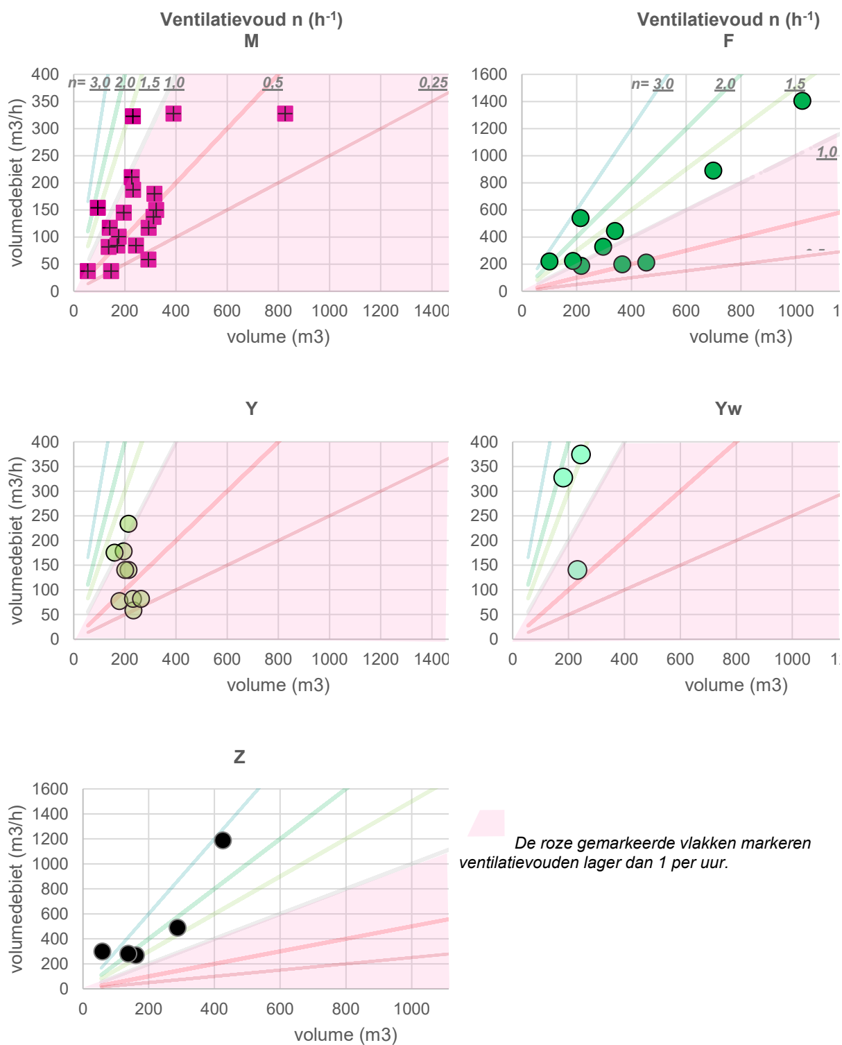
Figuur 17a,b,c,d,e Het ventilatievoud ( n per uur) ( \text{m}^3/\text{h} : \text{m}^3 ) voor alle onderzochte MUS-gebouwen ( n=0,25 \dots 3 \text{ h}^{-1} )
