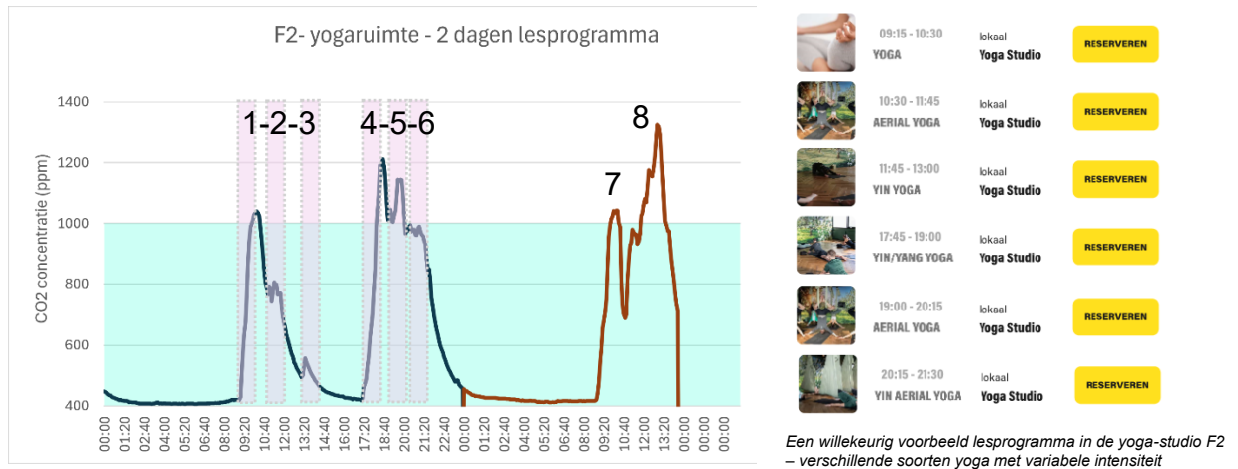
Figuur 32 De programmering en aard van de lessen, aantal aanwezigen, en de hoeveelheid ventilatie tijdens en na de lessen heeft invloed op het verloop van de CO 2 -concentratie in lesruimtes
